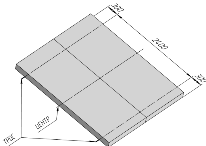
Рисунок 2 – Закладка тросов
