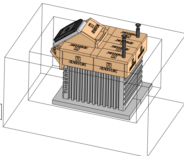
Рисунок 5 – Утепление погреба и закрепление тросами
